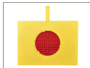
CTA100 Targhetta con catadiotro per fissaggio alle maglie della catena. Dimensioni: 140x105 mm.
