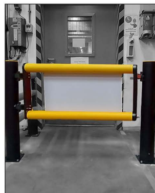
VLG150 Palo per cancello in polietilene. Colore nero. Altezza: 1000 mm. Diametro palo: 140 mm.
